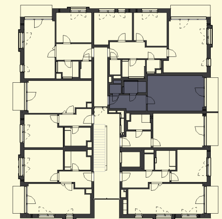
Půdorys podlaží / Floor Plan
